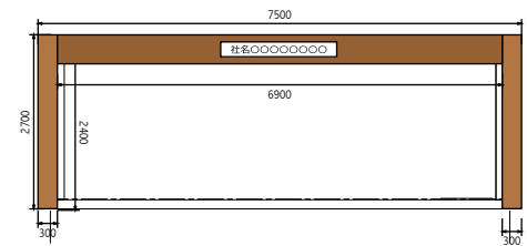
◎立面図(2小間)
