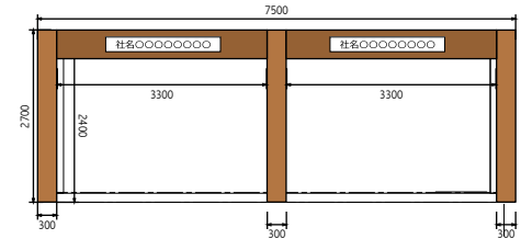
◎立面図(1小間)
