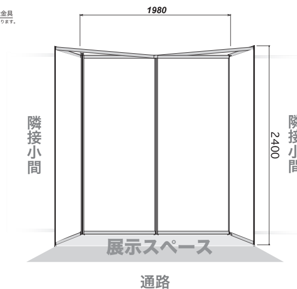
立面図 ※アイライン
