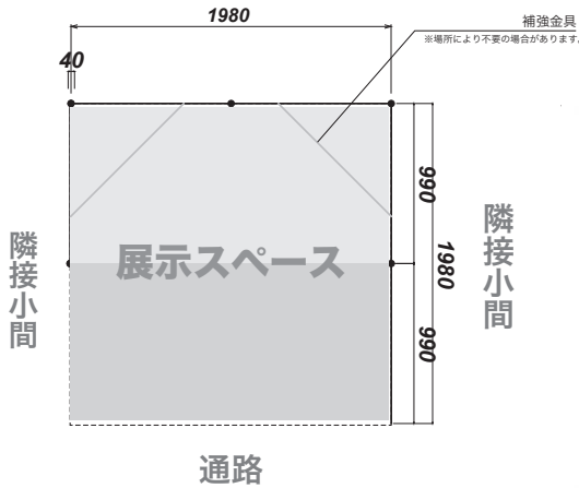
小間平面図
