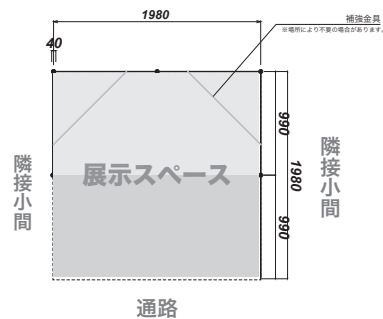
小間平面図
